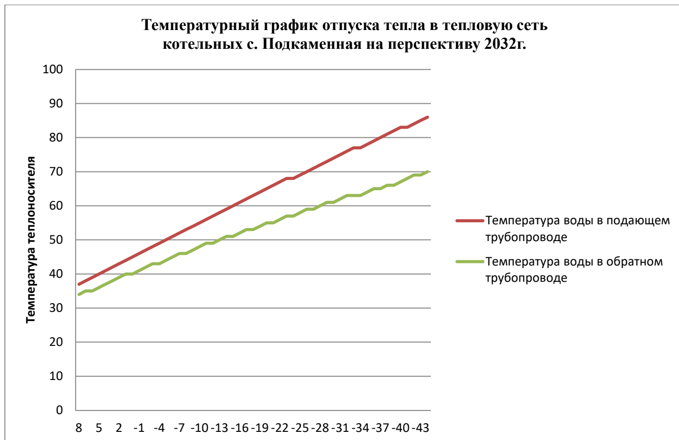
Рис. 1. Температурный график отпуска тепла от котельных п. Подкаменная на перспективу 2032г.
