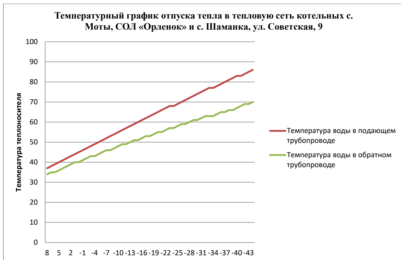
Рис. 1. Температурный график отпуска тепла от котельных с. Моты, СОЛ «Орленок» и с. Шаманка, ул. Советская, 9А на перспективу 2032г.
