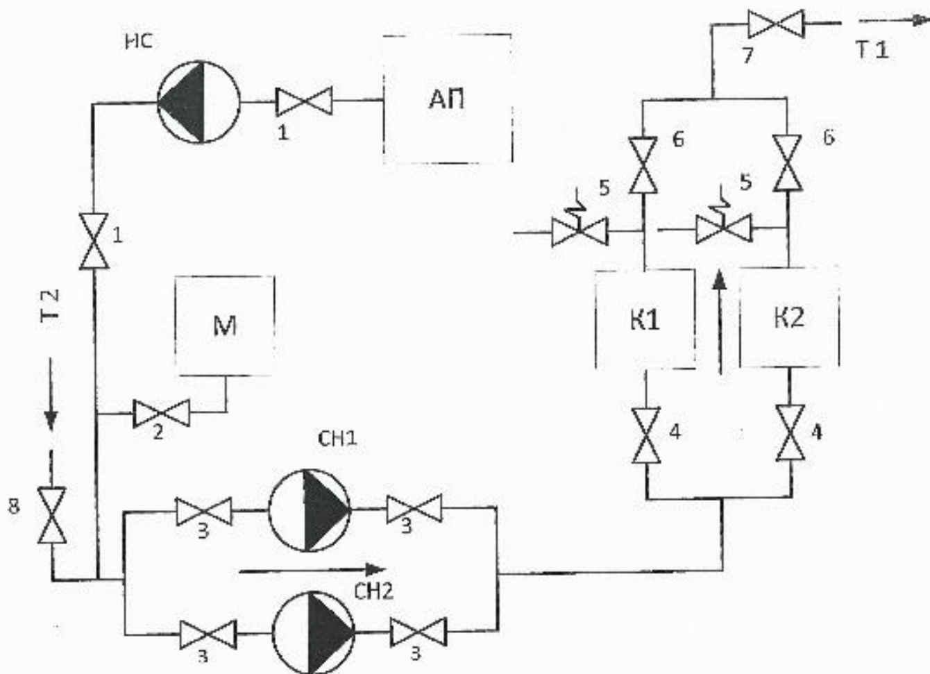
Рис. 2. Принципиальная схема котельной пер. Геологов, 1
