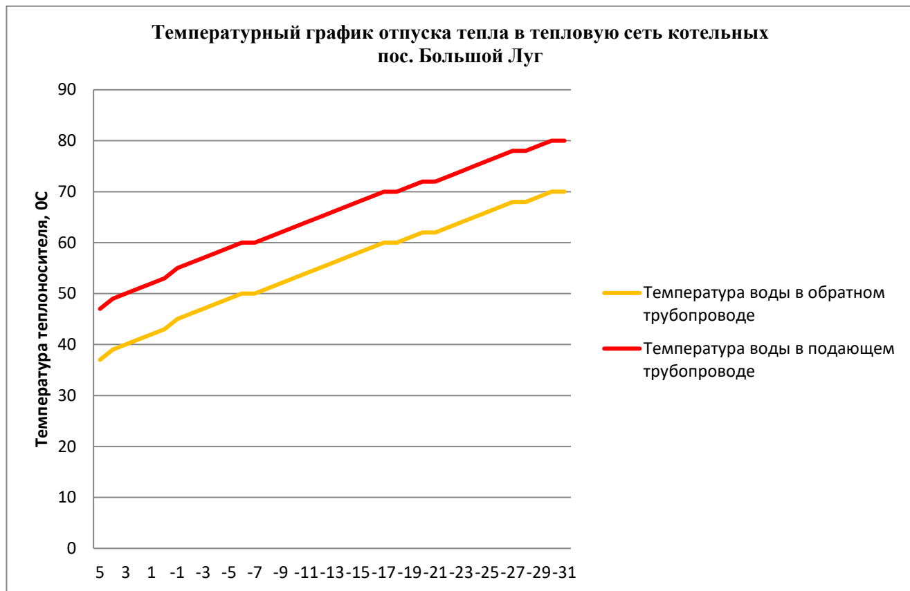
Рис. 1. Температурный график отпуска тепла от котельных Большого Луга.
